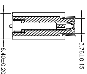
A-A SECTION
